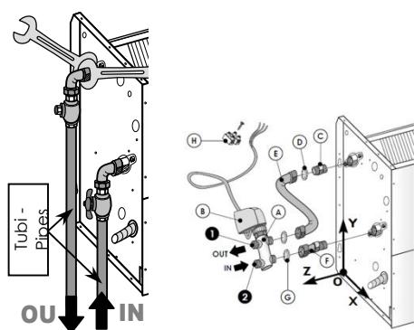
Attacchi idraulici dell'unità Ø ½" gas femmina Units water connections Ø ½" female gas
