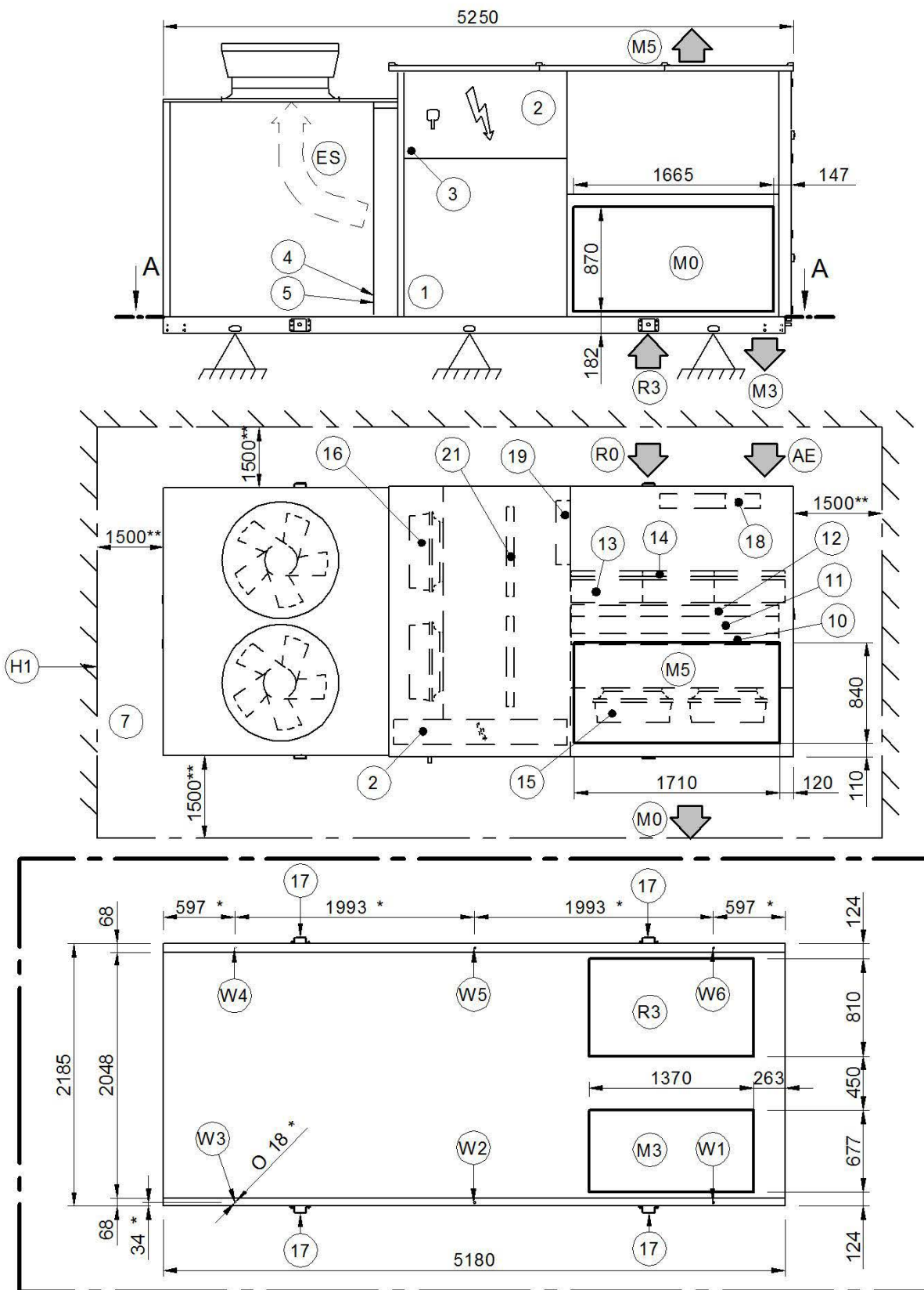
Sez A-A
