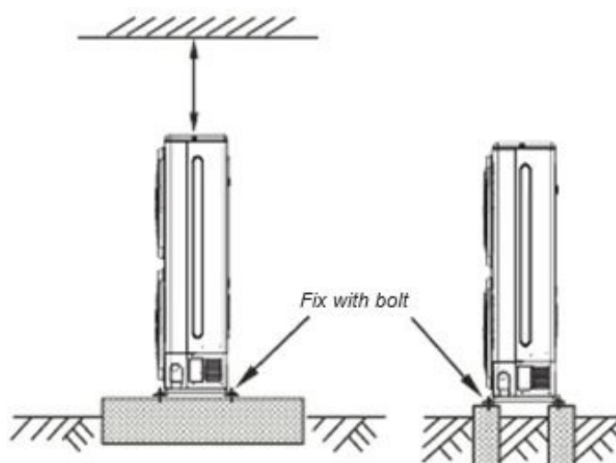
Figura 2.7: progetto strutturale di una comune base in cemento destinata ad un'unità esterna [mm]
